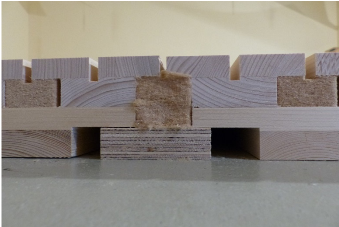
Bild 1: Querschnitt mit Detailansicht Plattenstoss
